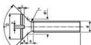
UNI 6109 - TSP - DIN 963 Art. 1300
