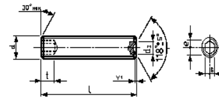
Art. 90 UNI 5929 / DIN 916
