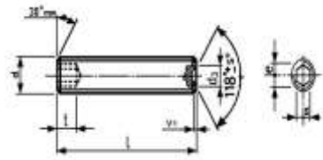
UNI 5929 DIN 916 Art. 1570
