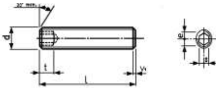
Art. 60 UNI 5923 / DIN 913
