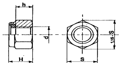
UNI 7473 - DIN 982 (alto)
