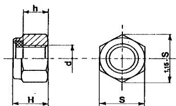
UNI 7473 - DIN 982 (alto)
