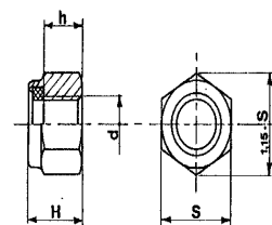
UNI 7474 - DIN -985 (basso)
