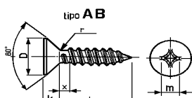
Art. 1110 UNI 6955 DIN 7982
