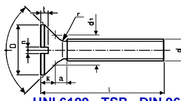
UNI 6109 - TSP - DIN 963 Art. 2410
