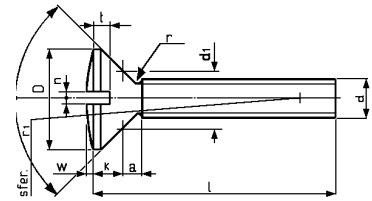
UNI 6110 - TSC - DIN 964 Art. 420
