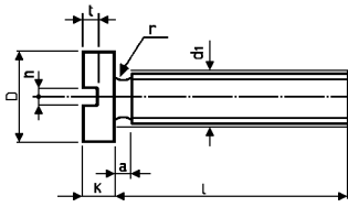
UNI 6107 - TC - DIN 84 Art. 400
